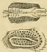
Fig. 747. Cythere Edwardsi Roem. sp. Miocän. Léognan bei Bordeaux. 22/1. (Nach Bosquet.)
