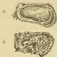
Fig. 748. Cythere Dunemelensis Norman. Pleistocän. Jordan Hill, England. a linke Schale von innen, b rechte Schale von aussen. Vergr. (Nach Brady.)
