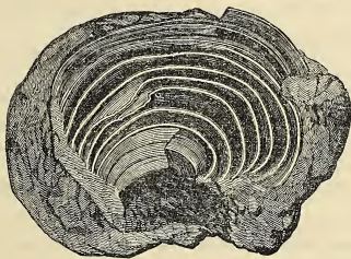
Astrocerium venustum.
